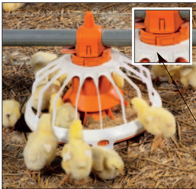
Кормушка FLUXX 360 с мелким днищем, заслонкой и решеткой из 16 ребер
